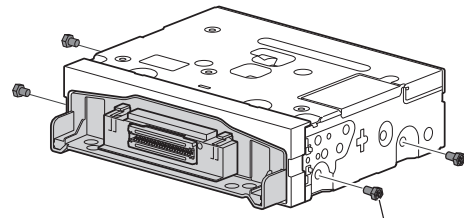
Sechskantschrauben (x4)
