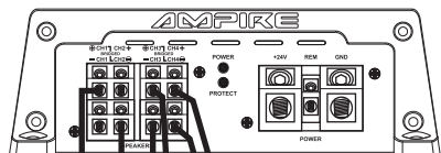
3-Kanal- Betrieb / 3- Channel Configuration
