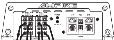
4-Kanal- Betrieb / 4- Channel Configuration
